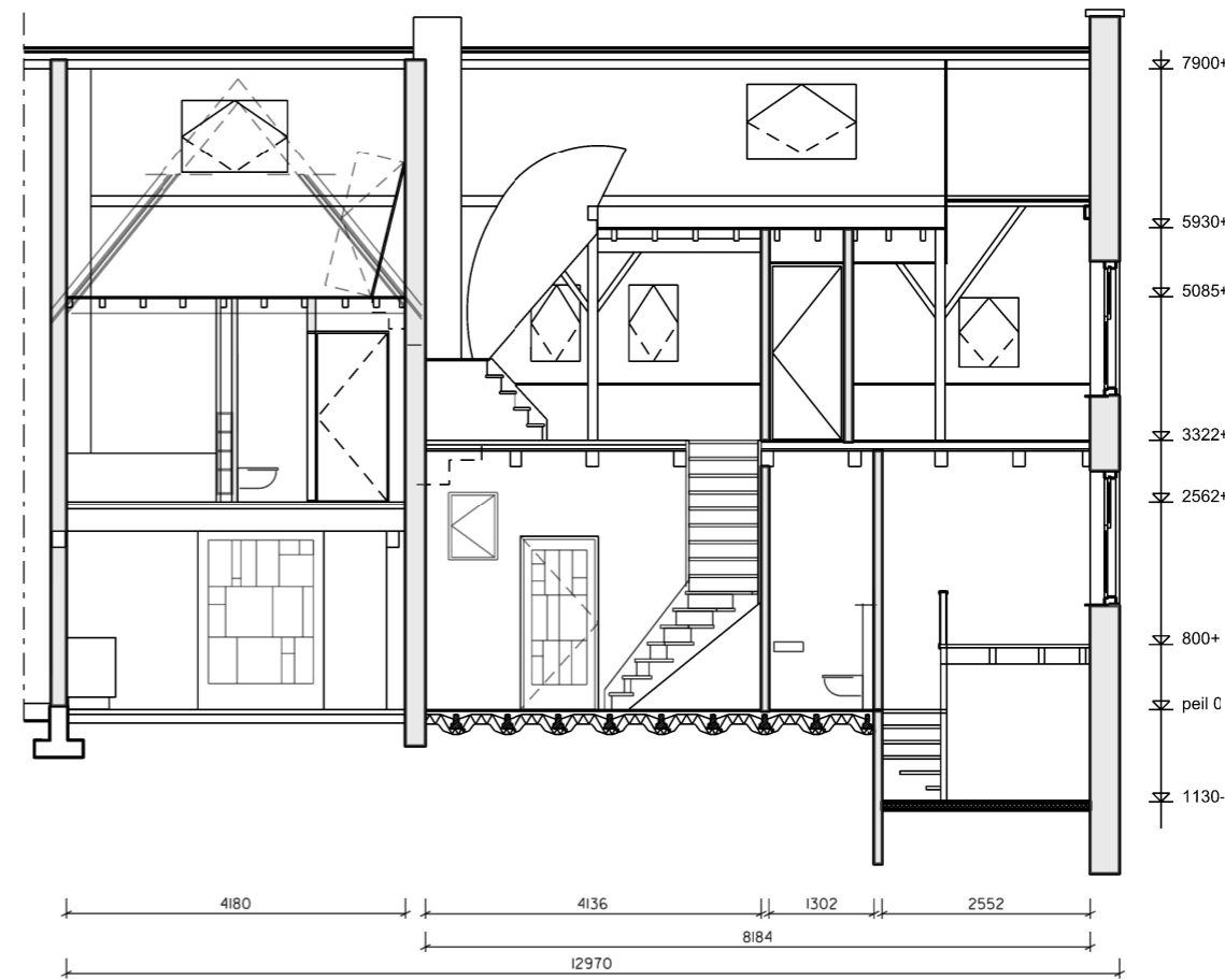
Doorsnede AA
